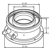
Адаптер для подключения дымохода Ø80/125 7716780184
