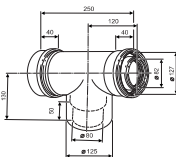
Коаксиальный отвод 90° с ревизионным люком, Ø80/125 7719002769
