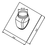
Накладка на дымовую трубу Ø80/125 для вертикального прохода через наклонную 25-45° крышу 7719002857
