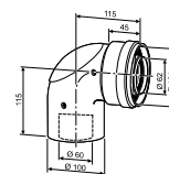
Коаксиальный отвод 90° с ревизионным люком, Ø60/100 7716050150
