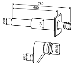
Двухтрубный горизонтальный комплект: удлинение 780 мм, Ø80/80 7716050081
