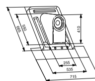
Накладка на дымовую трубу Ø100/150 для горизонтального прохода через наклонную 40-60° крышу 7719001031
