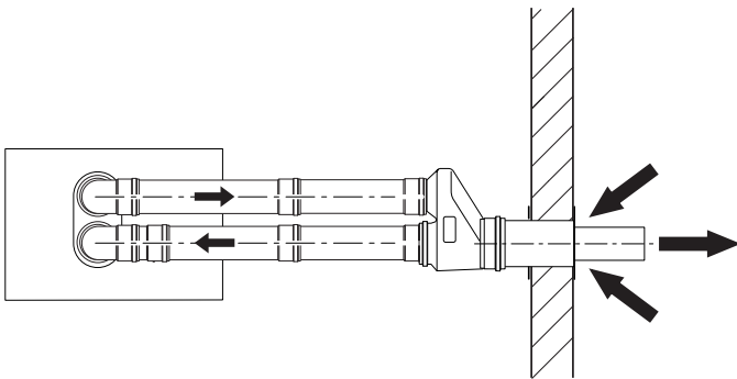
Рис. 10 Раздельное дымоотведение по С12/С13
