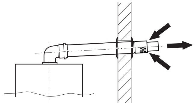
Рис. 11 Концентрическое дымоотведение по С12х/С13х
