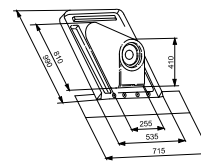
Накладка на дымовую трубу Ø100/150 для горизонтального прохода через наклонную 30-45° крышу 7719001028
