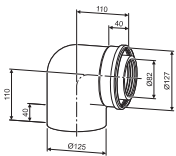
Коаксиальный отвод 90°, Ø80/125 7719002766
