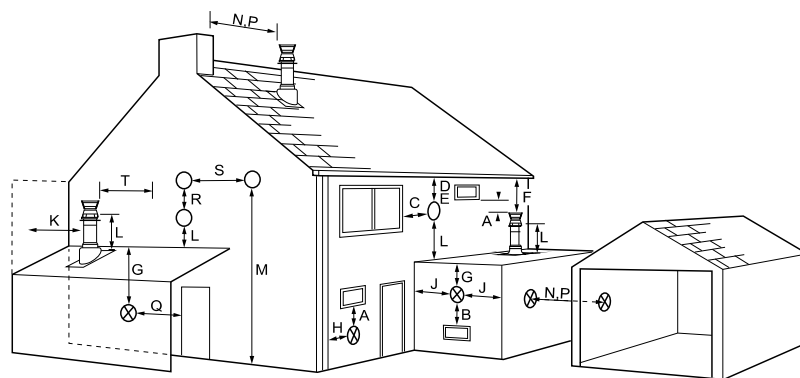
Рис. 6 Определение положения трубопровода отвода дымовых газов снаружи здания относительно наружных конструктивных элементов здания
