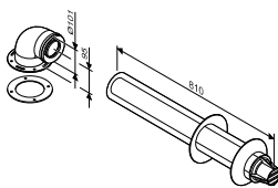
Коаксиальный горизонтальный комплект: отвод 90° + удлинение 810 мм, Ø60/100 7716050064
