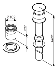
Коаксиальный вертикальный комплект: адаптер подключения к котлу + удлинение 1465 мм, Ø60/100 7716050071
