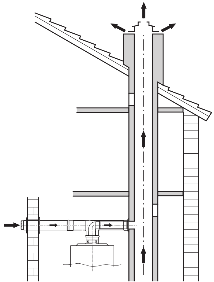
Рис. 21 Концентрическое дымоотведение по C82x/C83x
