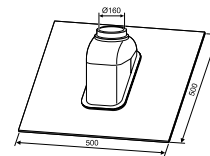
Накладка на дымовую трубу Ø100/150 для вертикального прохода через наклонную 25-45° крышу 7719002858
