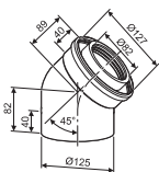
Коаксиальный отвод 45°, Ø80/125 7719002767
