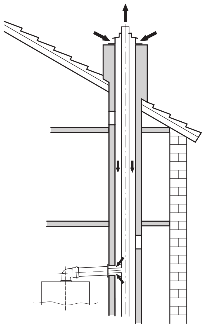
Рис. 15 Концентрическое дымоотведение по C42x/C43x
