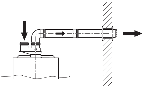
Рис. 7 Горизонтальное дымоотведение по В22/В23
