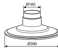
Накладка на дымовую трубу Ø100/150 для вертикального прохода через плоскую крышу 7719001657
