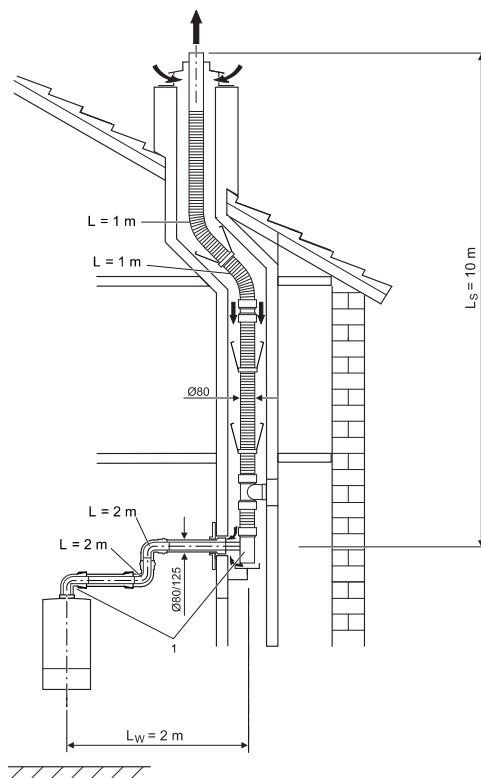
Рис. 22 Графическое представление монтажной ситуации
