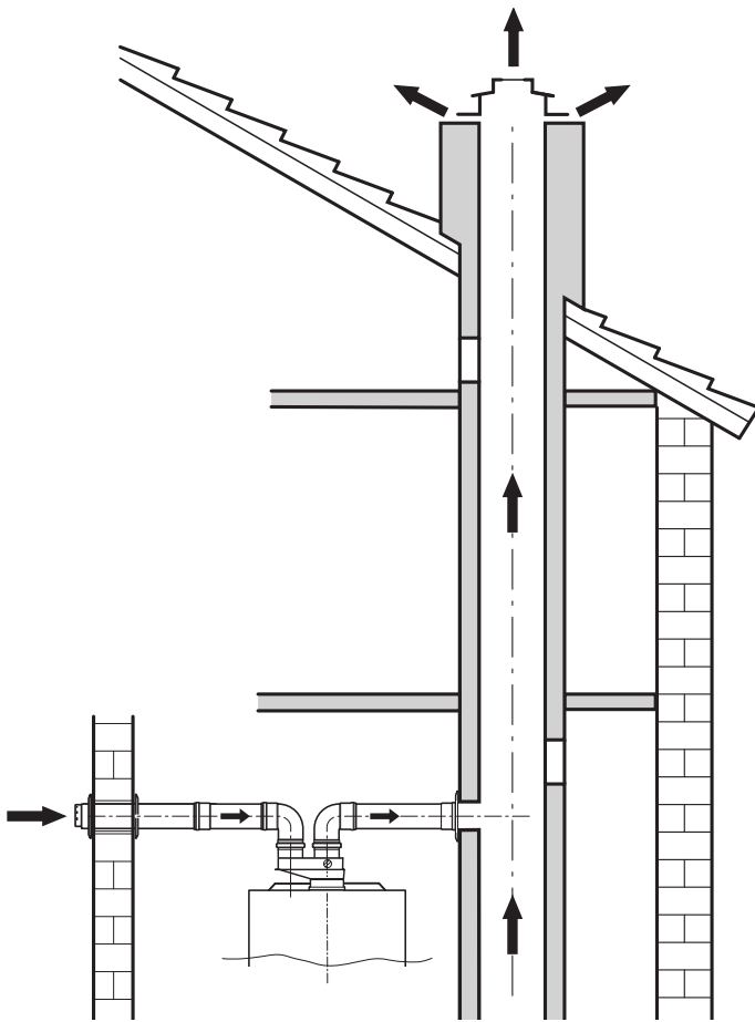
Рис. 20 Раздельное дымоотведение по C82/C83
