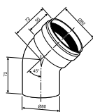
Отвод 45°, Ø80 7716050084
