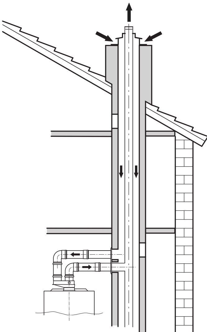
Рис. 14 Раздельное дымоотведение по C42/C43
