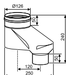
Адаптер для подключения раздельных дымоходов Ø80 к коаксиальному дымоходу Ø80/125 7716050082
