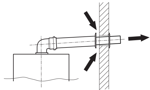
Рис. 9 Горизонтальное дымоотведение по В32/В33
