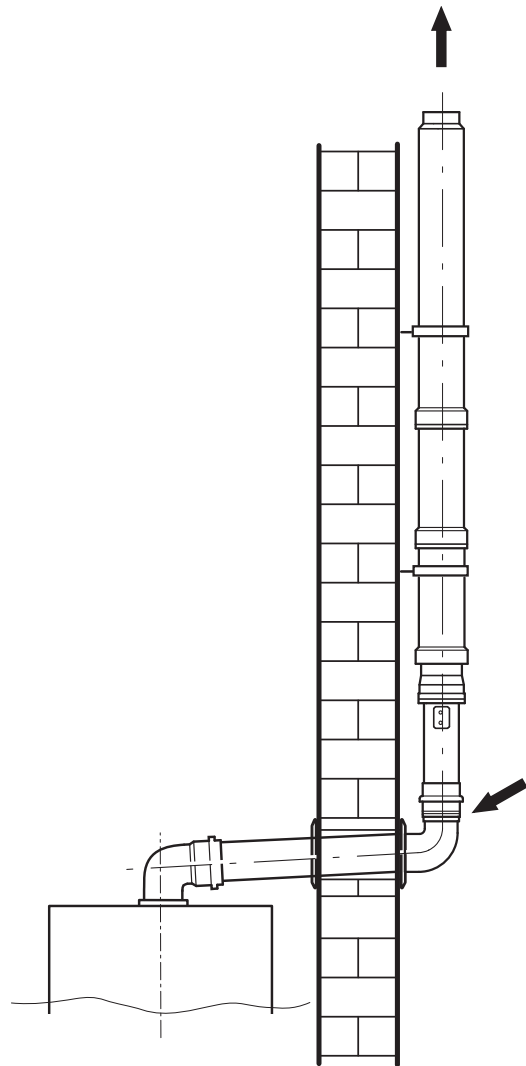
Рис. 17 Концентрическое дымоотведение по C52x/C53x
