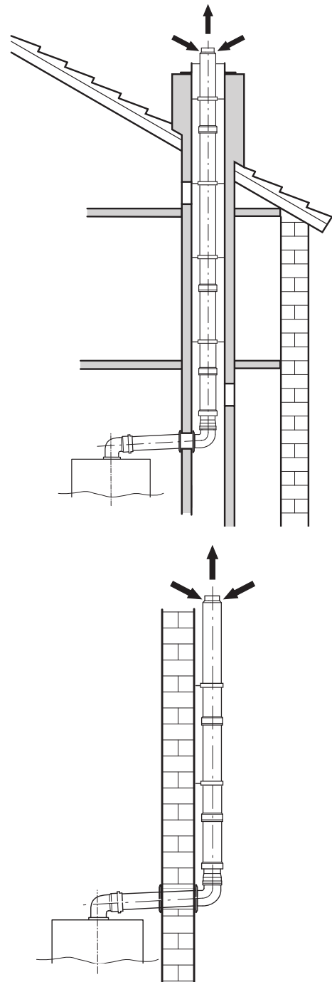
Рис. 19 Концентрическое дымоотведение по C62x/C63x
