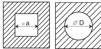
Рис. 1 Форма сечения шахты дымохода
