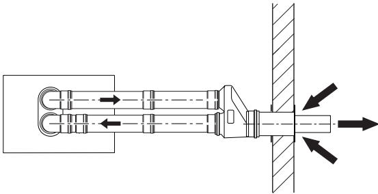
Рис. 3 Раздельные трубопроводы: подача воздуха на горение – по воздухопроводу; отвод продуктов сгорания – дымовой трубе
