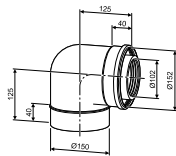
Коаксиальный отвод 90°, Ø100/150 7719002788
