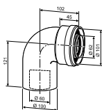
Коаксиальный отвод 90°, Ø60/100 7716050068
