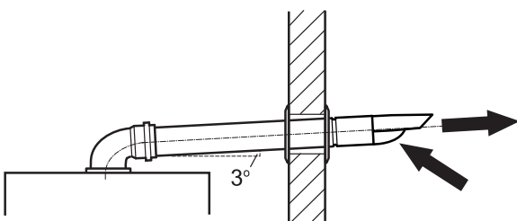
Рис. 4 Для конденсационных котлов монтаж дымовой трубы необходимо выполнять с подъемом 3° (5,2 см на метр трубы) в сторону движения дымовых газов (для отвода конденсата в сторону котла)
