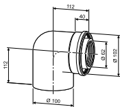
Коаксиальный отвод 90°, Ø60/100 7747210022
