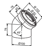
Коаксиальный отвод 45°, Ø60/100 7747210021
