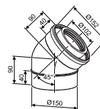
Коаксиальный отвод 45°, Ø100/150 7719002789
