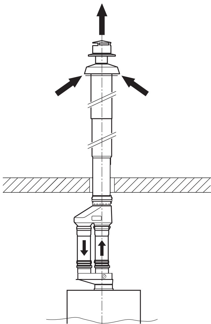
Рис. 12 Раздельное дымоотведение по C32/C33
