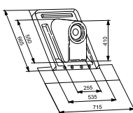
Накладка на дымовую трубу Ø80/125 для горизонтального прохода через наклонную 40-60° крышу 7719001031
