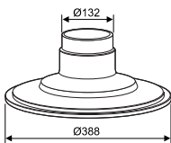
Накладка на дымовую трубу Ø80/125 для вертикального прохода через плоскую крышу 7719000838
