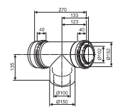
Коаксиальный отвод 90° с ревизионным люком, Ø100/150 7719002790
