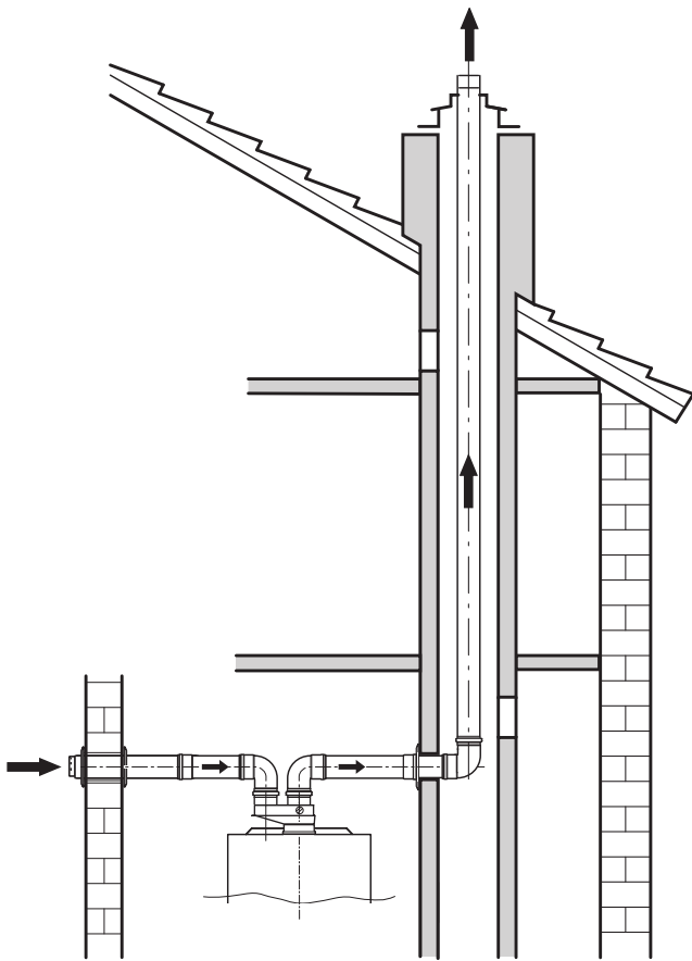
Рис. 18 Раздельное дымоотведение по C62/C63
