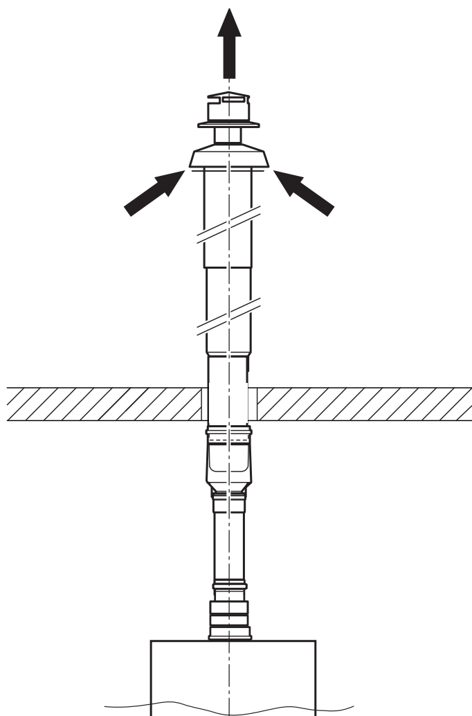
Рис. 13 Концентрическое дымоотведение по C32x/C33x
