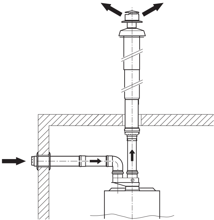
Рис. 16 Раздельное дымоотведение по C52/C53
