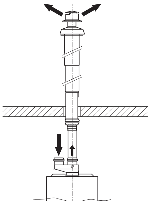
Рис. 8 Вертикальное дымоотведение по В22/В23
