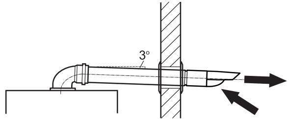
Рис. 5 Для конвекционных котлов монтаж дымовой трубы необходимо выполнять с уклоном 3° (5,2 см на метр трубы) в сторону движения дымовых газов (для отвода конденсата от котла)
