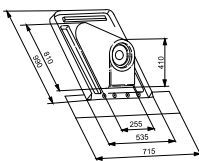
Накладка на дымовую трубу Ø80/125 для горизонтального прохода через наклонную 30-45° крышу 7719001028
