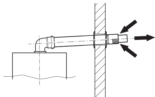
Рис. 2 Концентрические трубопроводы: подача воздуха на горение по внешней трубе; отвод продуктов сгорания – по внутренней трубе
