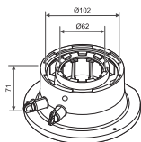
Адаптер для подключения дымохода Ø60/100 к Ø80/125 7719003381
